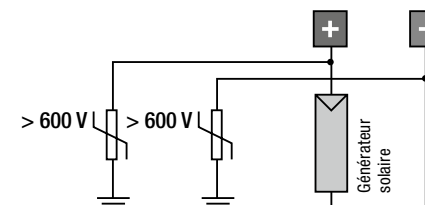
Le schéma ci-contre montre le raccordement de limiteurs de surtension du côté courant continu.
